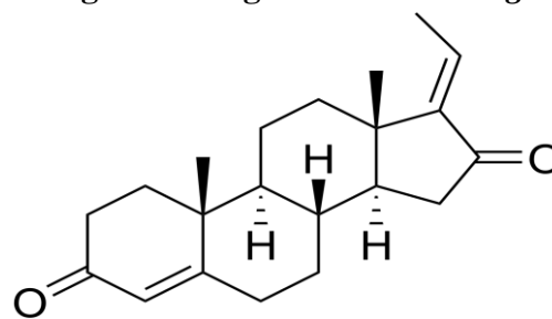
Fig.3 Guggulsterone - E
